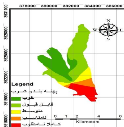
شکل ۷: نقشه پهنه‌بندی منطقه میان جنگل از لحاظ آب شرب
