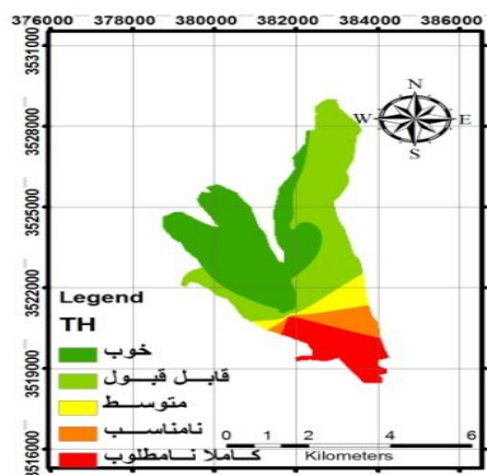
شکل ۶: نقشه هم ارزش TH منطقه میان جنگل فسا
