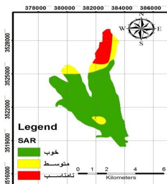
شکل ۹: نقشه هم ارزش SAR
