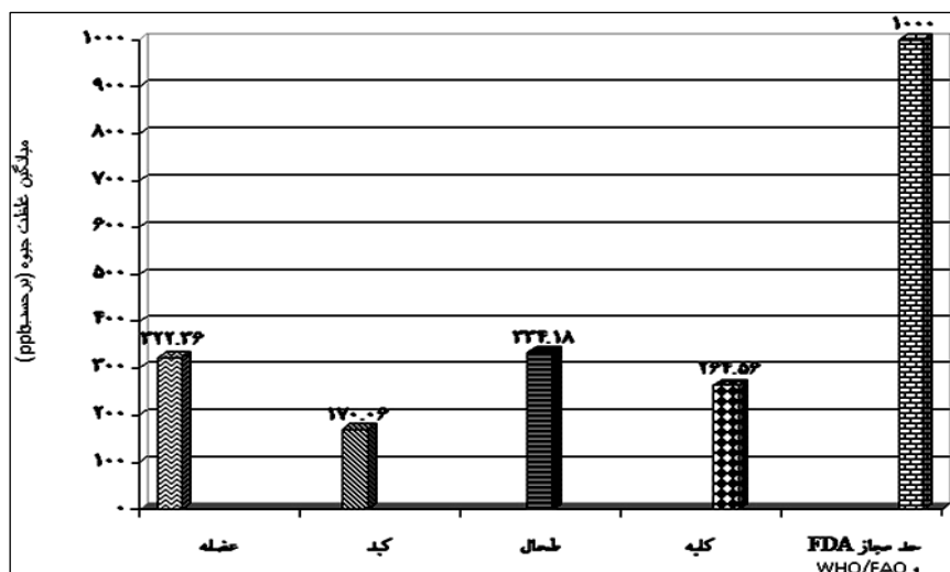
شکل ۳: مقایسه غلظت جیوه (ppb) در اندام‌های مختلف اردک‌ماهی ( Esox lucius ) تالاب انزلی (در سال ۱۳۹۱) با حد مجاز FDA و WHO/FAO.
