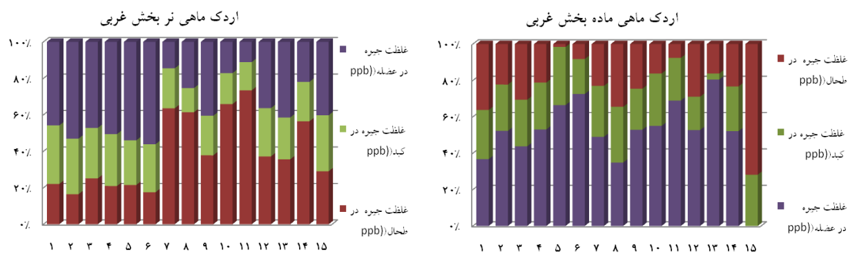
شکل ۱: مقایسه غلظت جیره (ppb) در بافت‌های مختلف اردک ماهی ( Esox lucius ) به کل جیره به تفکیک جنسیت و محل حضور در ۱۳۹۱.
