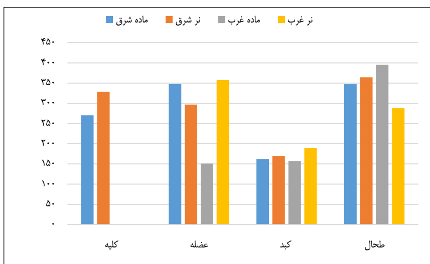
شکل ۲: مقایسه میانگین غلظت جیره (ppb) در اندام‌های مختلف اردک ماهی ( Esox lucius ) تفکیک جنسیت و محل حضور در ۱۳۹۱.
