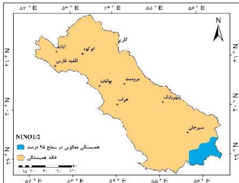
شکل ۹: همبستگی متوسط دمای حوضه ابرقو - سیرجان و الگوی Nino1.2 در ماه دسامبر.
