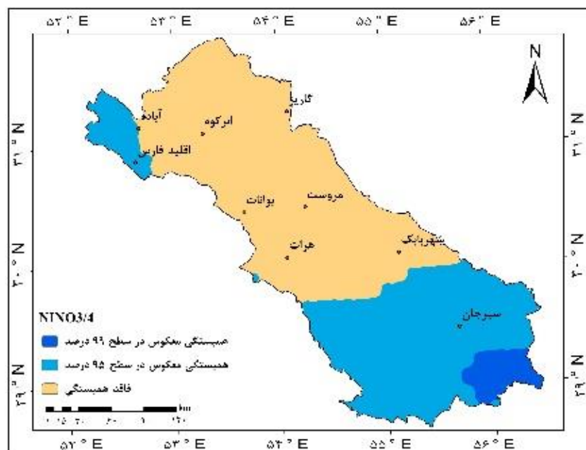
شکل ۱۰: همبستگی متوسط دمای حوضه ابرقو - سیرجان و الگوی Nino3.4 در ماه دسامبر.
