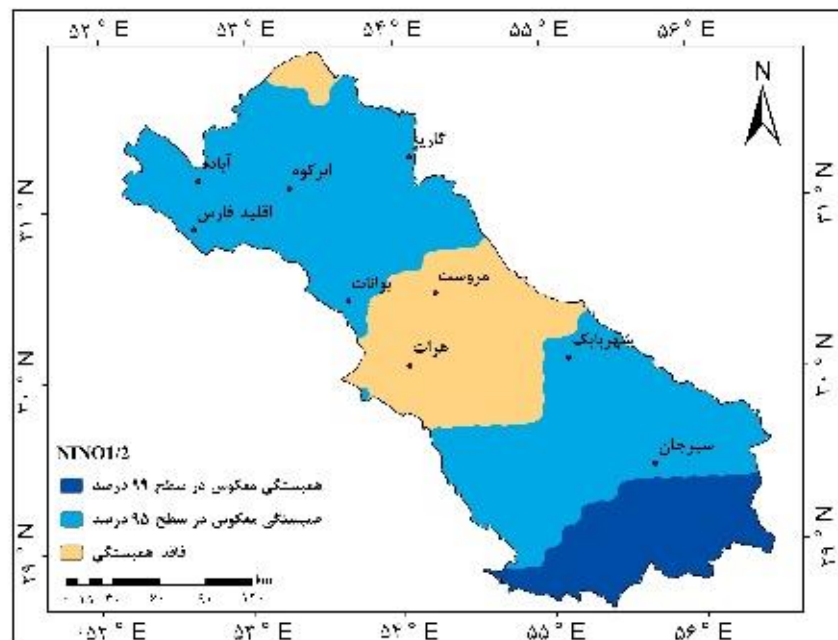
شکل ۶: همبستگی متوسط دمای حوضه ابرقو - سیرجان و الگوی Nino1.2 در ماه نوامبر.
