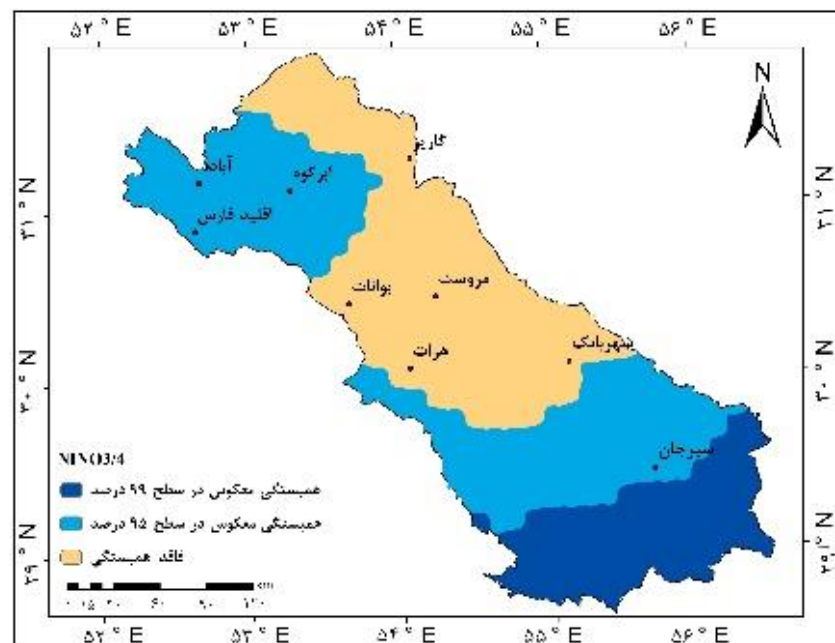
شکل ۷: همبستگی متوسط دمای حوضه ابرقو - سیرجان و الگوی Nino3.4 در ماه نوامبر.
