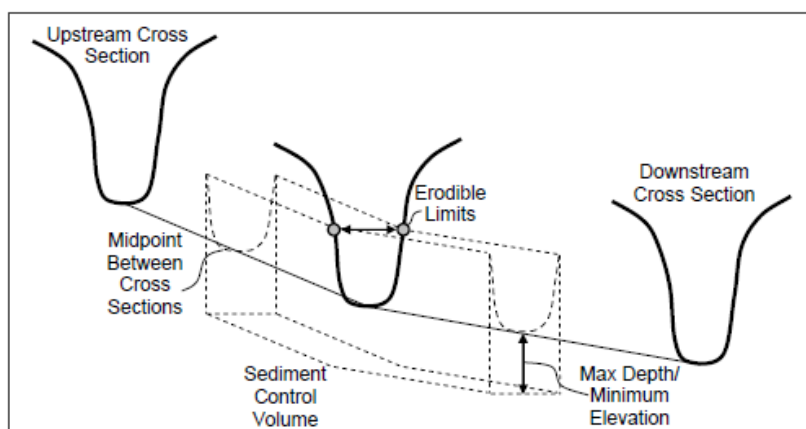
شکل ۴: شماتیکی از حجم کنترل رسوب برای یک مقطع عرضی (USACE, 2022)
