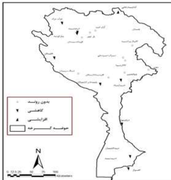
شکل ۵: پراکنش مکانی ایستگاه‌ها با روندهای افزایشی (▲)، کاهشی (▼) و بدون روند (○) با سطح معنی‌داری بالای ۵ و ۱۰ درصد برای سری‌های زمانی بارش سالانه در دوره آماری ۲۰۱۱-۱۹۷۱ در حوضه کرخه.
