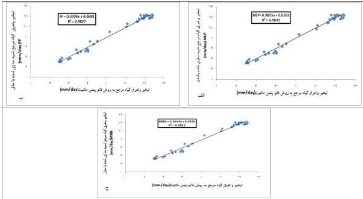
شکل ۵: مقایسه تبخیر و تعرق گیاه مرجع محاسبه شده با روش فائو پنمن مانتهیت با سه شبکه MLP (الف)، FF (ب) و MNN (ج) در سناریو دوازدهم.
