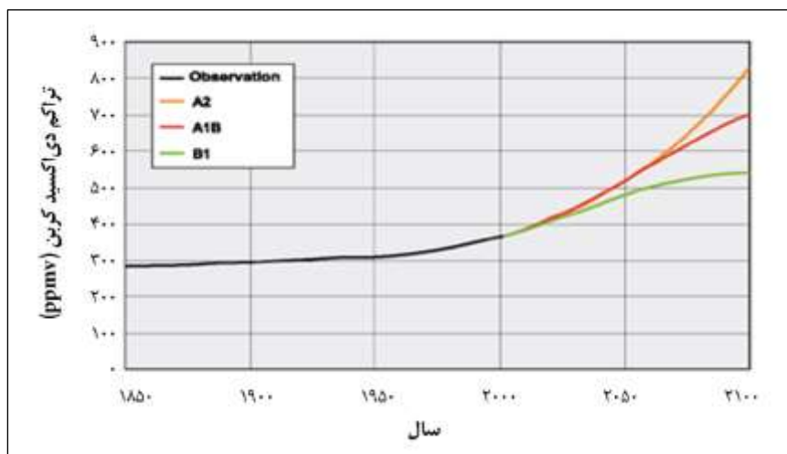
شکل ۳: نمودار میزان روند تغییرات میزان دی اکسید کربن موجود در جو طی دوره زمانی (۲۱۰۰-۱۸۵۰) (Roeckner et al., 2006).
