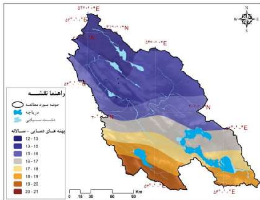
شکل ۵: پهنه‌های دما سالانه بر اساس سناریوی A1B
