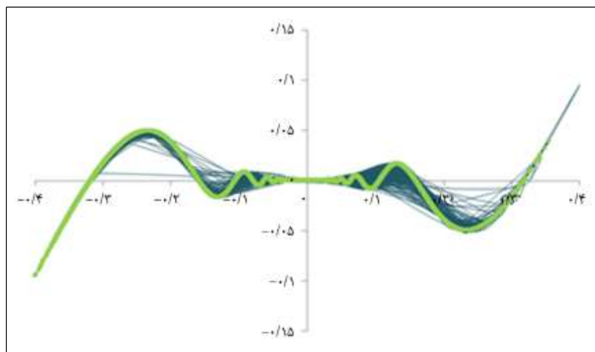
شکل ۱۸: ساختار بر خالی روزانه فراسنج پیش بینی شده دما نقطه دوم.
