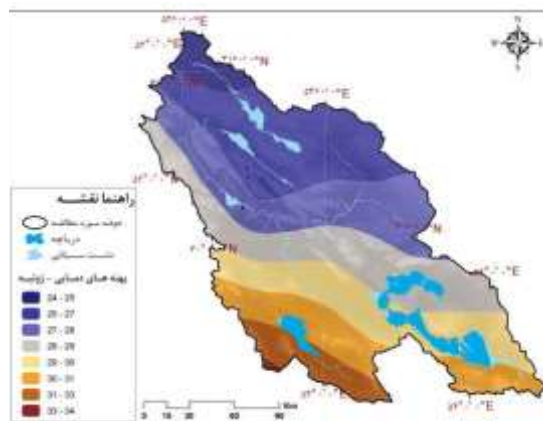
شکل ۱۲: پهنه‌های دما در ماه ژوئیه بر اساس
