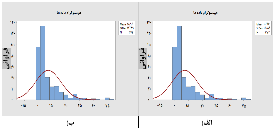
شکل ۳: الف) هستوگرام داده‌های نرمال شده، ب) هستوگرام داده‌های واقعی.
