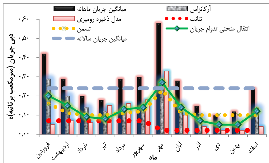
شکل ۴: مقادیر میانگین جریان ماهانه، میانگین جریان سالانه و جریان زیست‌محیطی برآورد شده رودخانه غاز محله به روش‌های مختلف.
