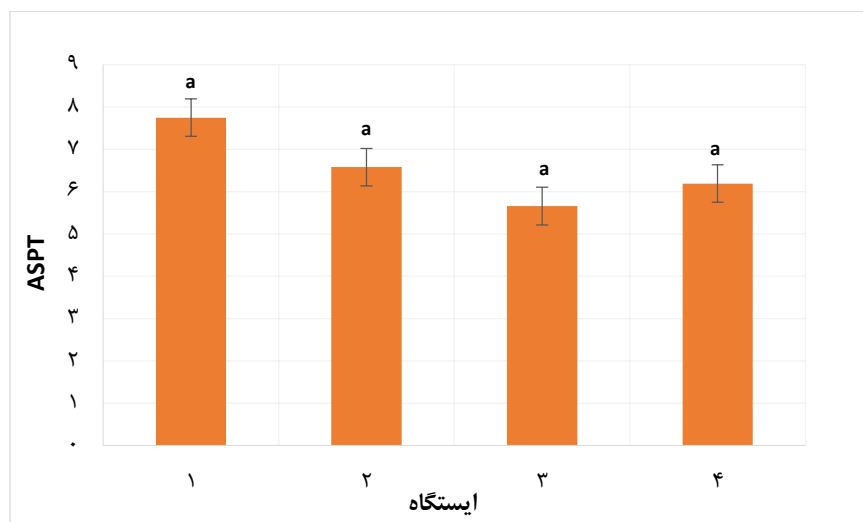
شکل ۴: تغییرات مقادیر شاخص ASPT (میانگین \pm انحراف معیار) در ایستگاه‌های منتخب تالاب هشیلان (فصل سرد، ۱۳۹۳).
