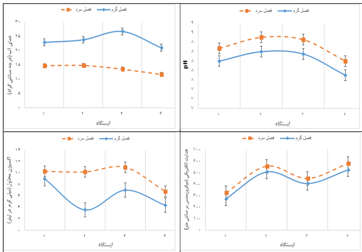
شکل ۳: نوسانات فاکتورهای فیزیکی و شیمیایی آب (دمای آب، اکسیژن محلول، هدایت الکتریکی و pH) (میانگین \pm انحراف معیار) در ایستگاه‌های منتخب تالاب هشیلان طی دو فصل (۱۳۹۳-۱۳۹۴).
