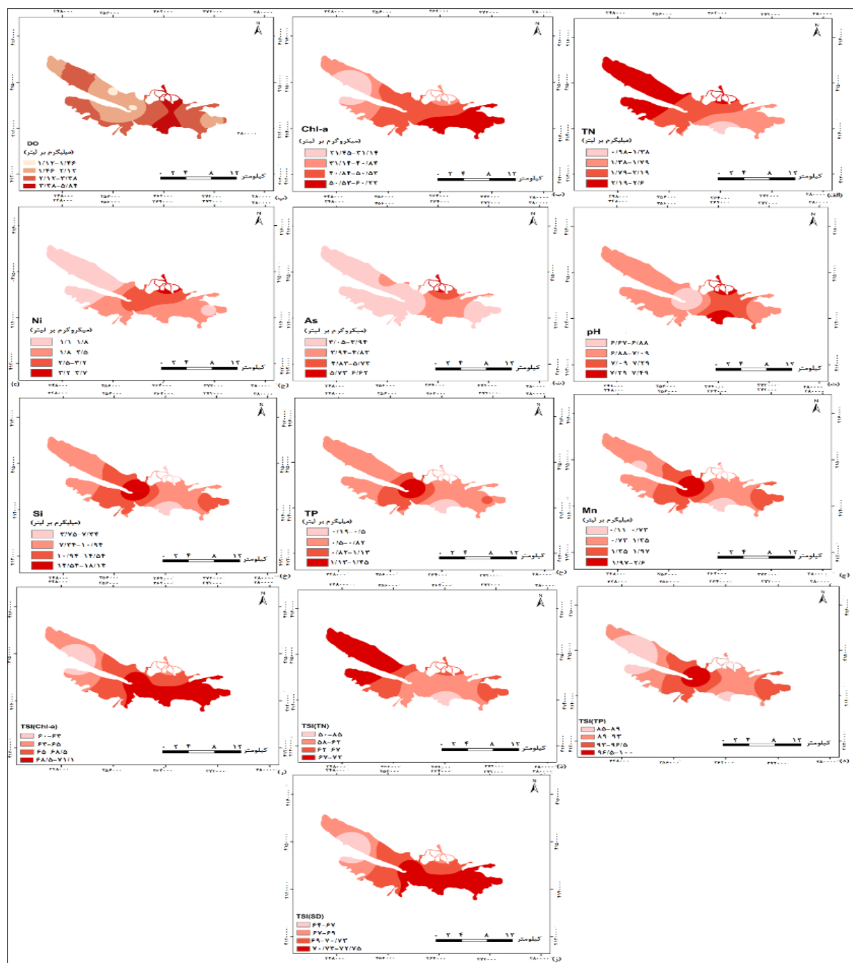
شکل ۳: پراکنش پارامترهای کیفی آب تالاب انزلی (الف TN (ب Chl-a (پ DO، ت pH (ث As (ج Ni (چ Mn (ح TP (خ Si (د TSI(TP) (ذ TSI(TN) (ر TSI(Chl-a) ؛ TSI(SD) برآورد شده توسط روش کریجینگ اصلاح شده در سال ۱۳۹۷.
