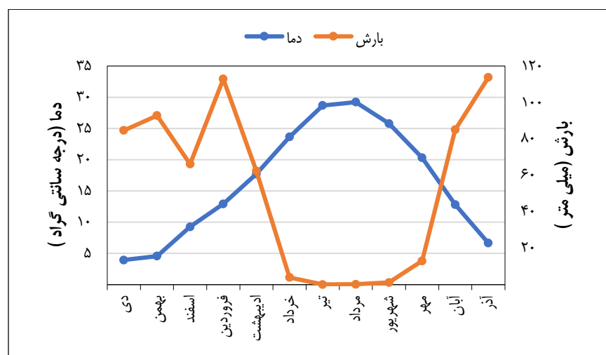
شکل ۵: منحنی آمبروترمیک ایستگاه سینوپتیک شهرستان دورود (۱۳۷۹-۱۳۹۷).
