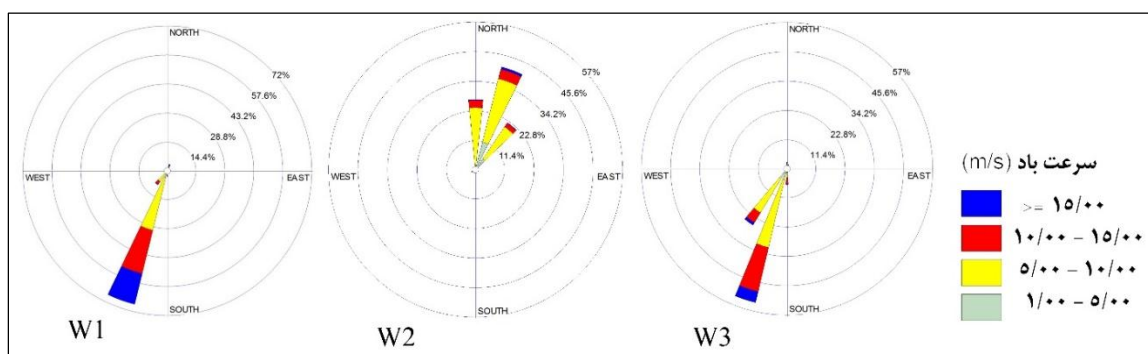
شکل ۶: گلباد ترسیم شده از محدوده تالاب‌های موردبررسی طی دوره ۱۸ ساله (۱۳۷۹-۱۳۹۷) W1: دریاچه گهر و تالاب تنوردر، W2: تالاب‌های پلدختر، W3: تالاب بیشه‌دالان).
