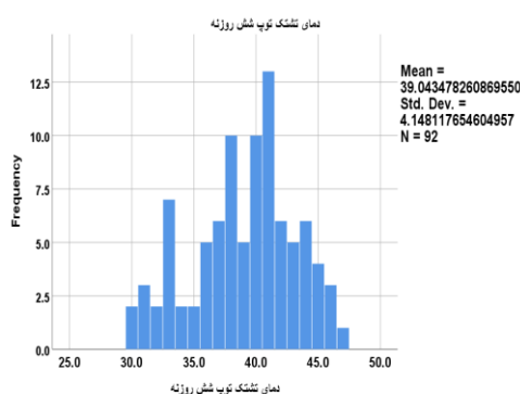
شکل ۶: هیستوگرام فراوانی نسبی دمای تشتک شاهد و تشتک دارای توپ.
