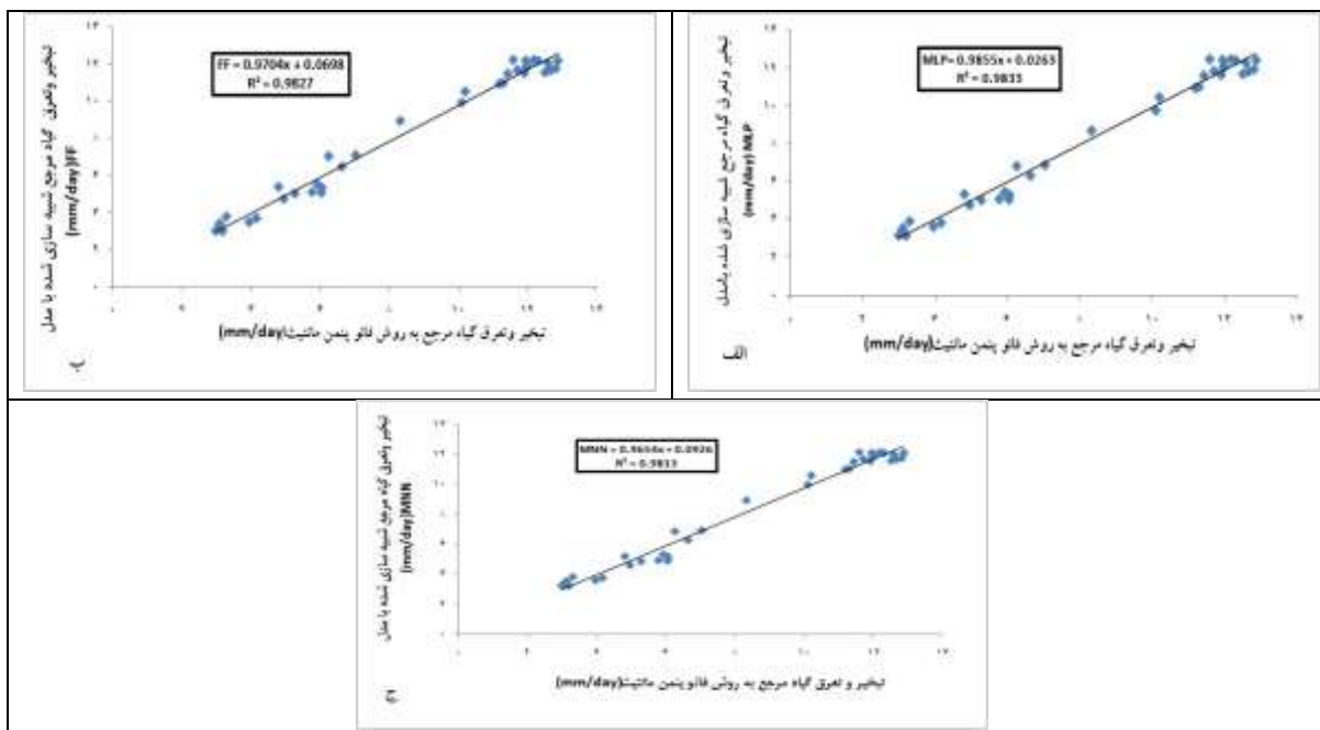
شکل ۵: مقایسه تبخیر و تعرق گیاه مرجع محاسبه‌شده با روش فائونین مانتیت با سه شبکه MLP (الف)، FF (ب) و MNN (ج) در سناریو دوازدهم.
