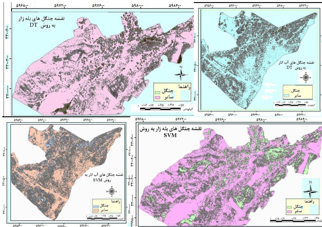
شکل ۳: نقشه عارضه جنگل با طبقه‌بندی بردار پشتیبان و درخت تصمیم به ترتیب از سمت راست جنگل‌های روستای به‌زار (سایت ۱)، جنگل‌های روستای انار (سایت ۲) (سال بررسی ۱۳۹۴).
