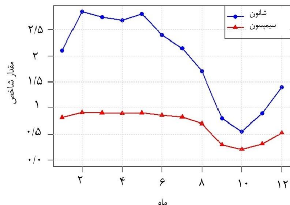
شکل ۱۰: نمودار شاخص‌های شانون و سیمپسون
