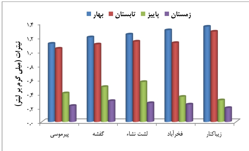
شکل ۷: تغییرات غلظت نیترات در ایستگاه‌های رودخانه اشک در فصول مختلف (۱۳۹۲-۱۳۹۱).
