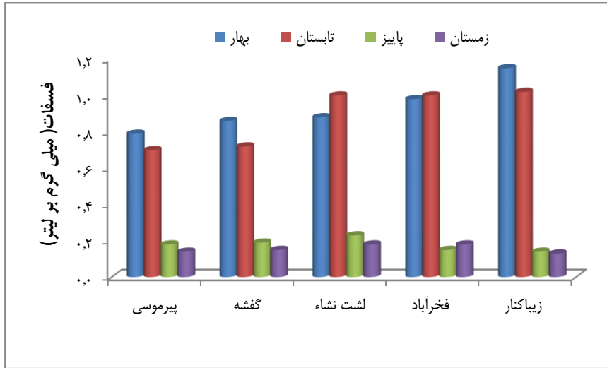
شکل ۶: تغییرات غلظت فسفات در ایستگاه‌های رودخانه اشک در فصول مختلف (۱۳۹۲-۱۳۹۱).
